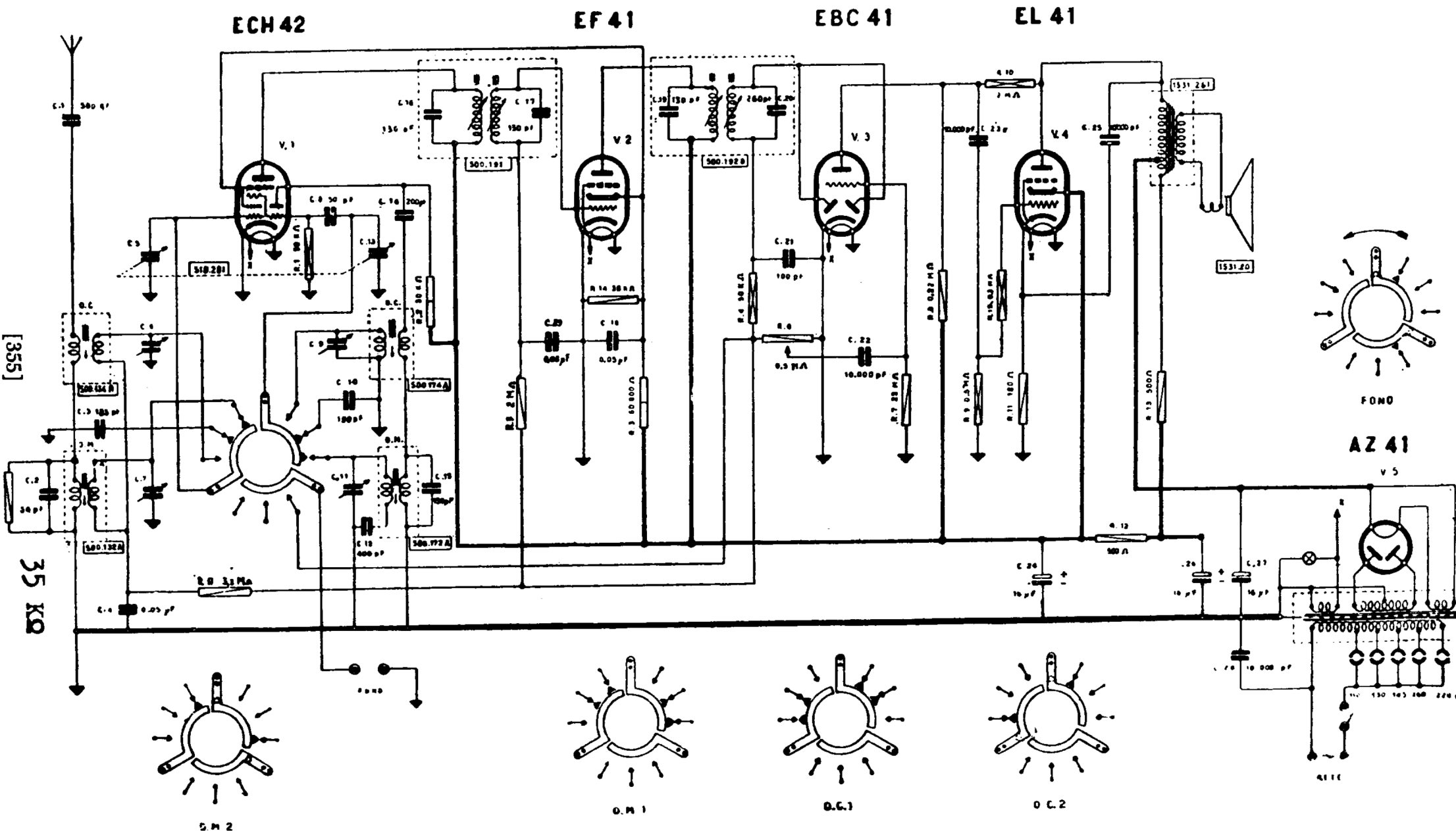
VOCE DEL PADRONE - Mod. Marconi 1531. Quattro gamme d'onda: OM1: 570-430 m; OM2: 435-187 m; OC1: 52-38,5 m; OC2: 38,5-18 m. Media frequenza 465 kc. Potenza d'uscita indistorta 3 watt. Consumo circa 45 watt.
